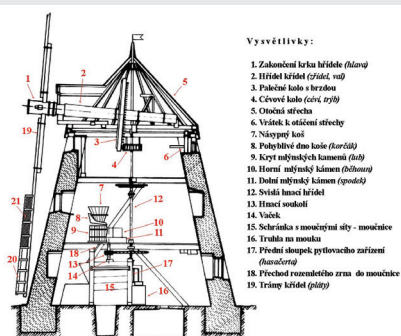
Konstrukce větrného mlýnu, zdroj: povetnik.cz
